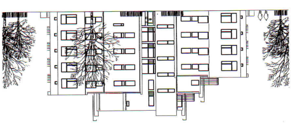
FASAD FRÅN NORDOST, HUS H
