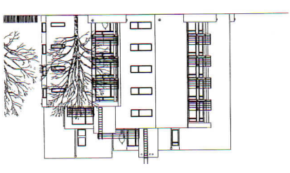
FASAD FRÅN SYDOST, HUS H
