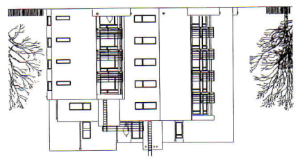
FASAD FRÅN SYDOST, HUS G
